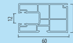
PG 08 Standaard geleider voor het CleverBox-systeem.
