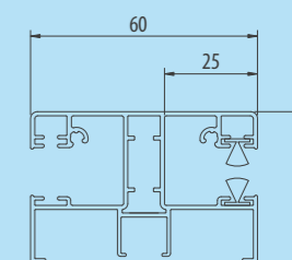
ALU PPDA 60/12 Het aluminium equivalent van de standaard geleider voor het Opoterm-systeem. Toegepaste schroeven - RD2
