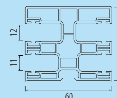
PG 09 Geleider voor rolgordijnen met ingebouwd vliegenraam.
