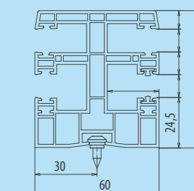
geleider R163 Geleider toegepast in rolgordijn met ingebouwd vliegenreem. Toegepaste schroeven - RD1
