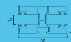
PG 02 Geleider voor rolgordijnen met onderverdeling.
