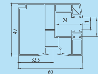
geleider R151 Standaard geleider EXTE EXAKT. Toegepaste schroeven - RD1
