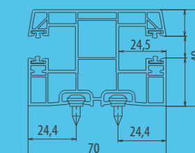
geleider R158 Geleider toegepast in rolgordijn met onderverdeling. Toegepaste schroeven - RD1
